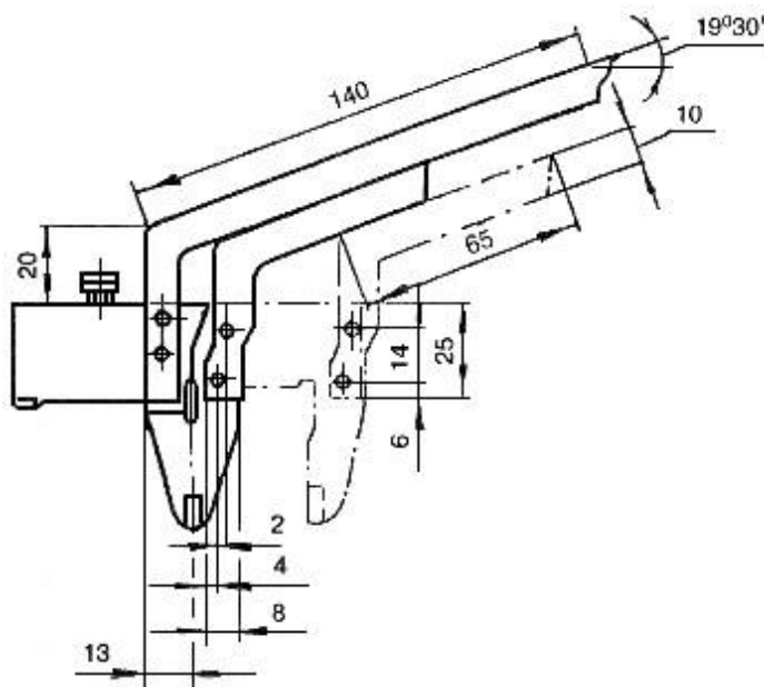
Рисунок 3 - Передвижной шаблон
